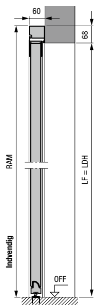
Separat dør med aluminium-standardkarm profiltipe 2 Montering bag åbningen
