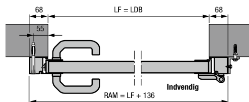
Separat dør med aluminium-standardkarm profiltipe 2 Montering bag åbningen
