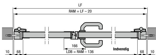
2-fløjet separat dør med aluminium-standardkarm profiltipe 2 Montering i åbningen
