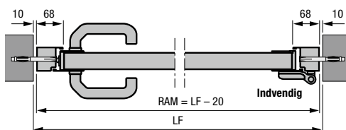
Separat dør med aluminium-standardkarm profiltipe 2 Montering i åbningen
