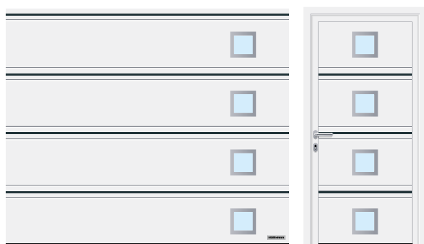
T-profilering (LPU 42), trafikavid RAL 9016, design indlægselement motif 501 og designelement motif 461 antracitgrå RAL 7016, separat dør med samme udseende
