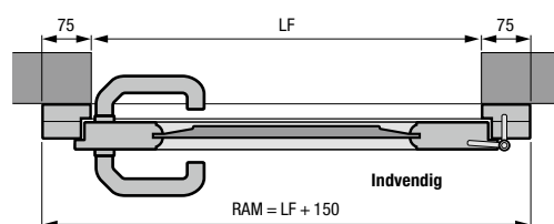
Separat dør i massivt træ Montering bag åbningen
