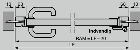
Separat dør med aluminiumstandardkarm, profiltipe 2 Montering i åbningen
