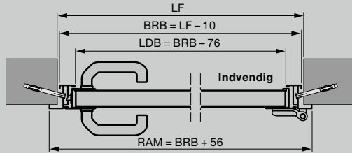
Separat dør med aluminiumhjørnekarm, profiltipe 1 eller 2 Indvendigt anslag
