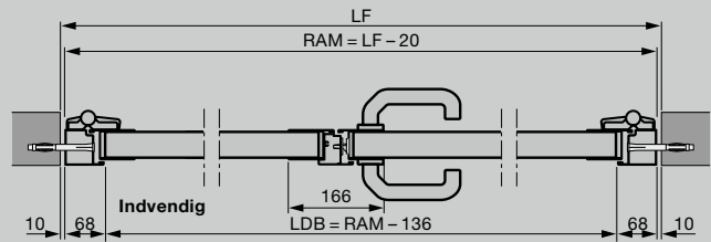
2-fløjet dør med aluminiumstandardkarm, profiltipe 2 Montering i åbningen
