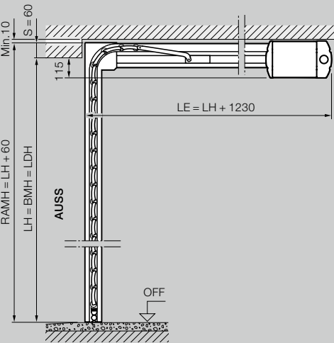
Størrelsesområde port med vandret skinneføring RollMatic OD*
