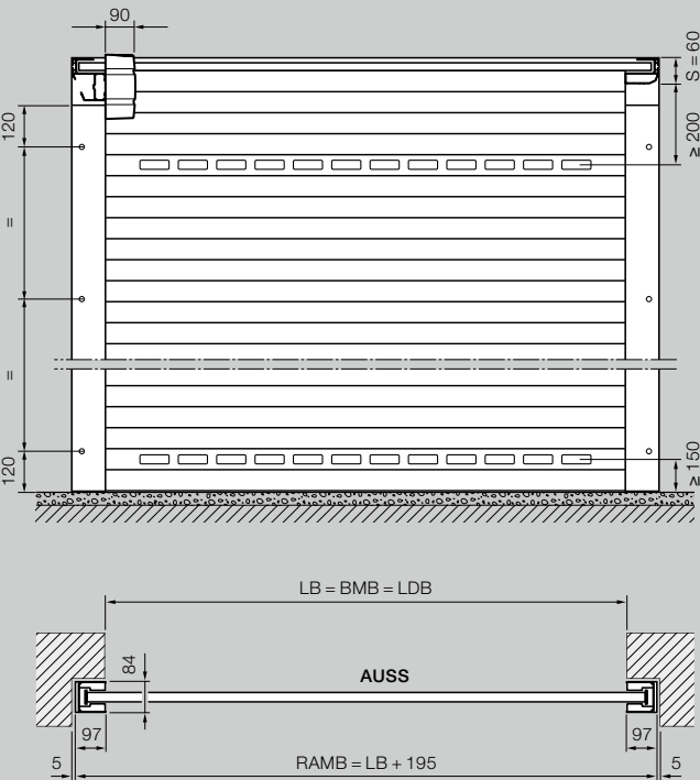
Rulleport med vandret skinneføring Montering bag åbningen, visning anslagsside
