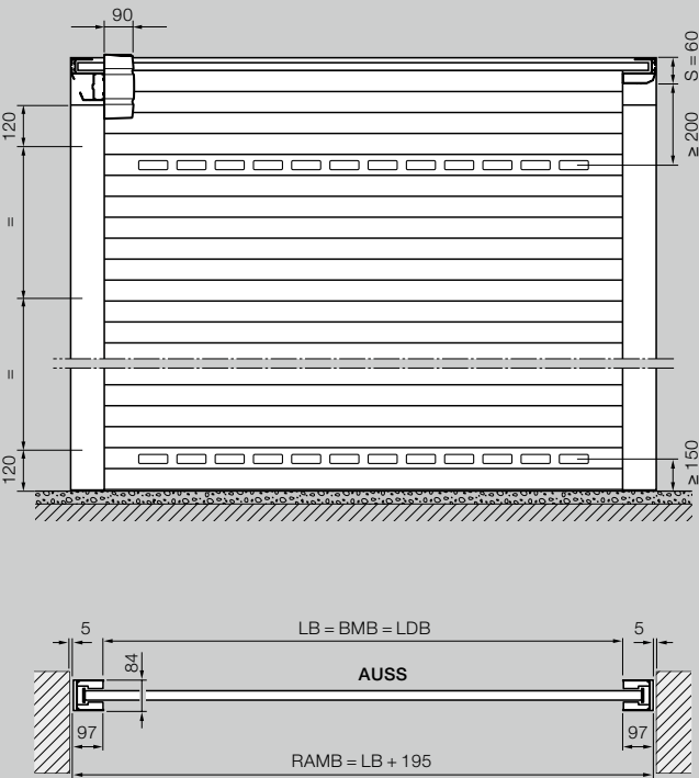
Rulleport med vandret skinneføring Montering i åbningen, set indefra
